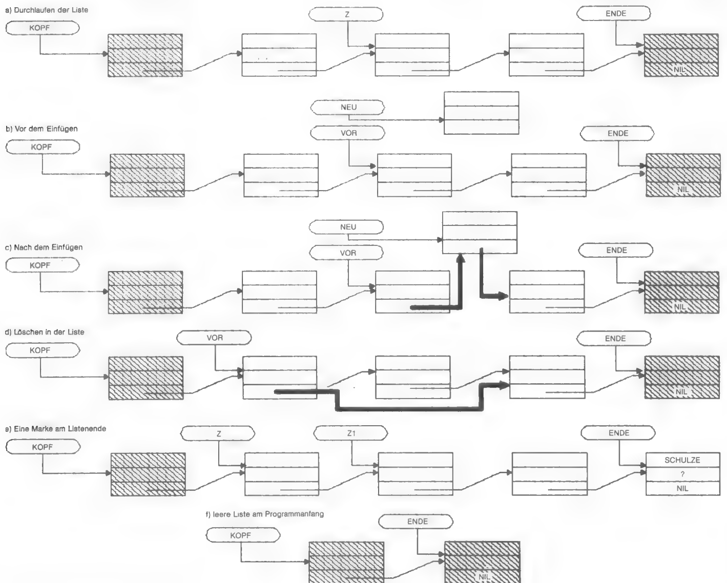
Bild 4. Die Kundenliste aus Listing 1
